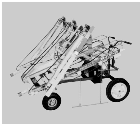
「BJX-2」を折りたたんだ状態
